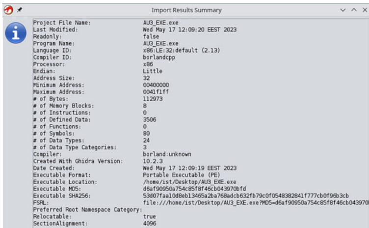
Рисунок 1 – Інформація щодо файлу, який було імпортовано в середовище ПЗ «Ghidra»
