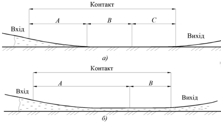
Рис. 1. Взаємодія шини автомобільного колеса з поверхнею дорожнього покриття, яка перебуває у вологому стані: а) аквапланування відсутнє; б) випадок аквапланування
