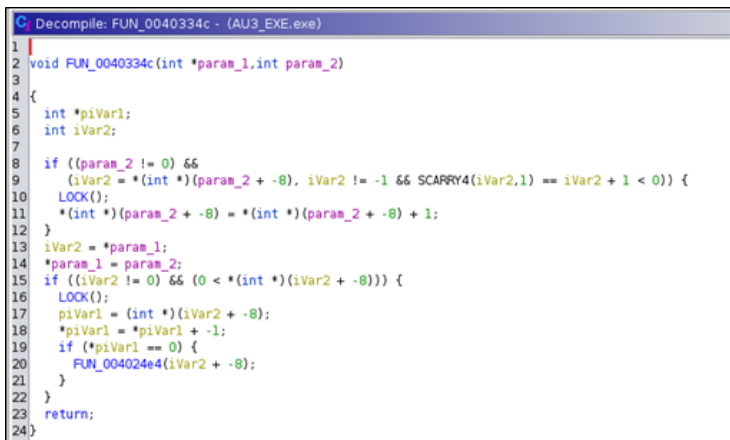
Рисунок 6 – Інформаційний вміст функції «FUN_0040334c»
