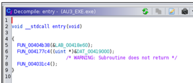
Рисунок 4 – Вміст функції «entry» при її перегляді у вікні декомпілятора
