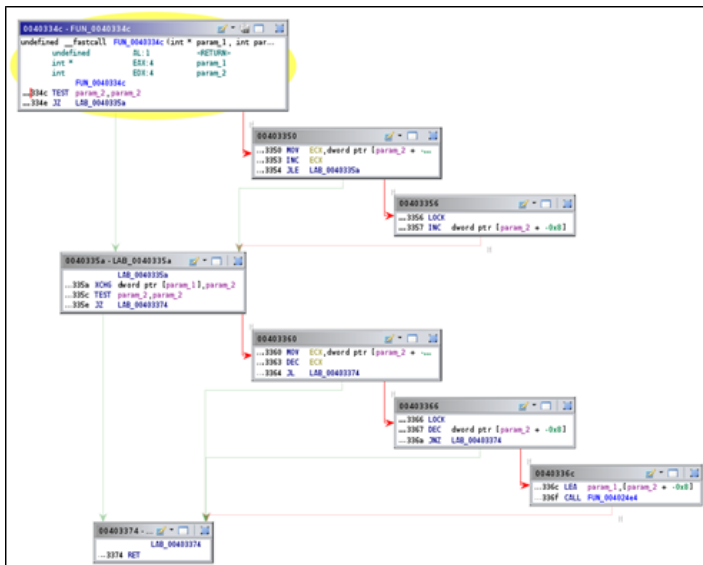
Рисунок 7 – Процес виконання функції «FUN_0040334c» у вигляді графу
