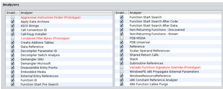
Рисунок 2 – Налаштування щодо аналізу для проведення зворотного програмування
