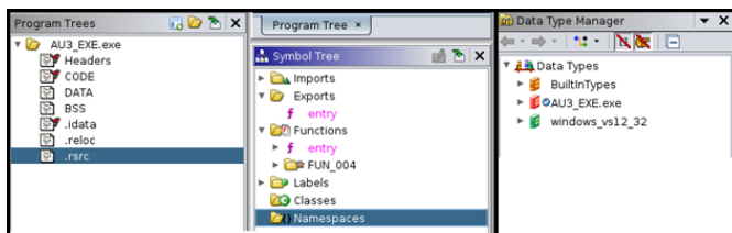
Рисунок 3 – Відображення результатів аналізу виконуючого файлу у вікнах «Program Trees», «Symbol Tree» та «Data Type Manager»
